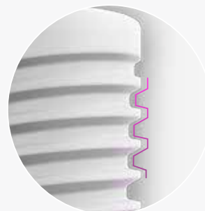
Design a doppia filettatura trapezoidale.
